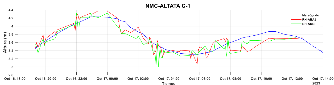
Figura 25. Comparativa de tendencia de alturas GNSS/Mareográficas respecto al tiempo, campaña uno.
