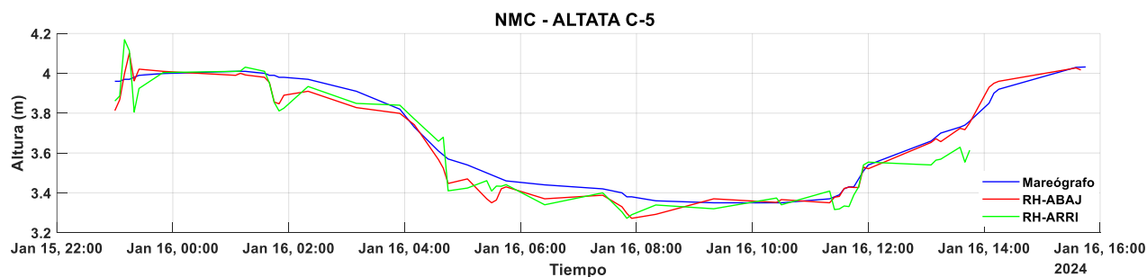
Figura 33. Tendencia de mediciones relativas del nivel del mar mediante GNSS-R y MC para la campaña cuatro.
