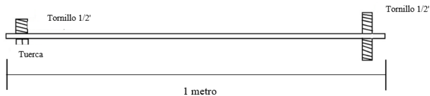
Figura 18. Representación esquemática de la solera (barra) para la toma de datos. Fuente: elaboración propia.
