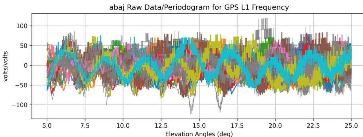
Figura 22. Periodograma SNR; representación gráfica sinusoidal de las señales GPS reflejas para en L1, estación: ABAJ.
