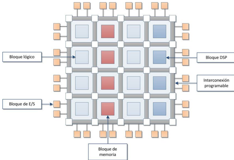
Figura 2-1.: Diagrama de la composición de un FPGA extraído de [39]
