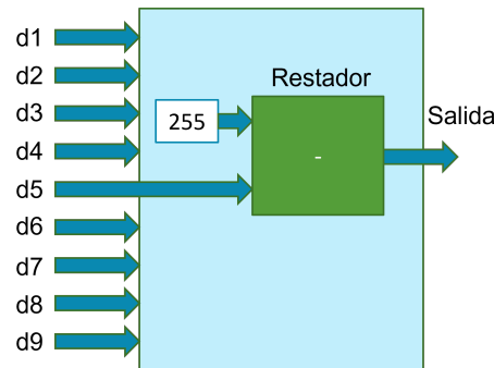
Figura 3-14.: Diagrama de la negación.
