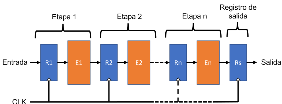
Figura 2-7.: Diagrama de una arquitectura de procesamiento.
