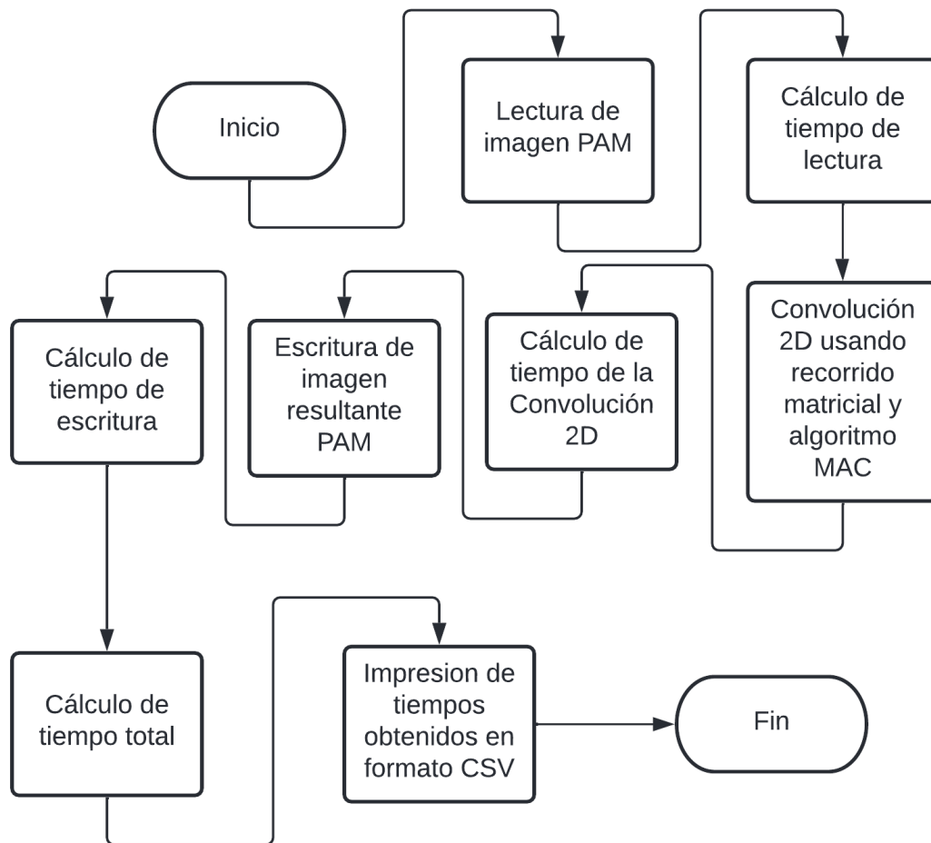
Figura 3-20.: Diagrama de flujo del software de la convolución 2D solo por software.
