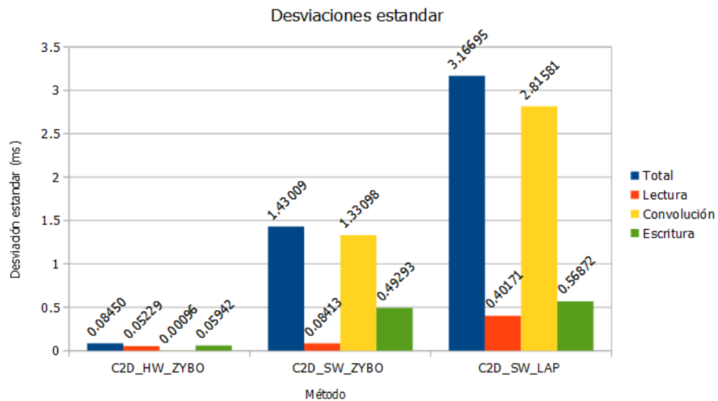
Figura 4-10.: Desviación estándar del tiempo necesario para calcular la convolución 2D.
