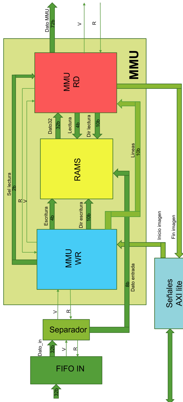
Figura 3-8.: Composición del MMU.
