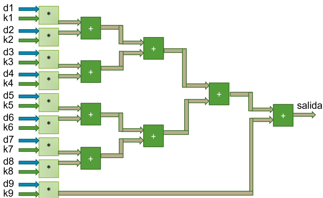
Figura 3-15.: Diagrama de la convolución.
