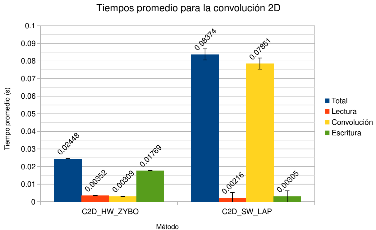
Figura 4-8.: Tiempos promedios para la convolución 2D en dos métodos.
