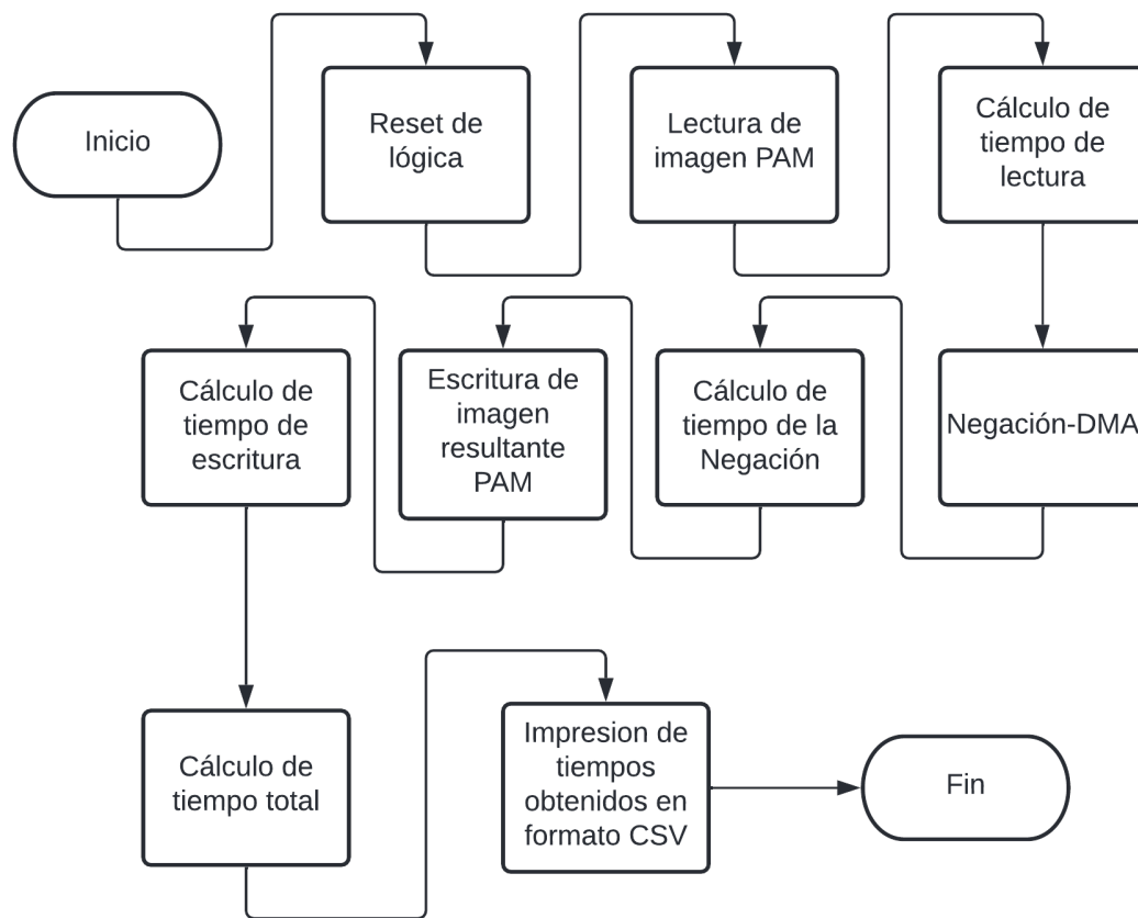
Figura 3-16.: Diagrama de flujo del software de interfaz de la negación por hardware.
