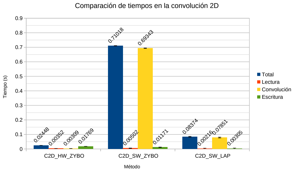
Figura 4-7.: Tiempos promedios de las tres implementaciones para la convolución 2D.
