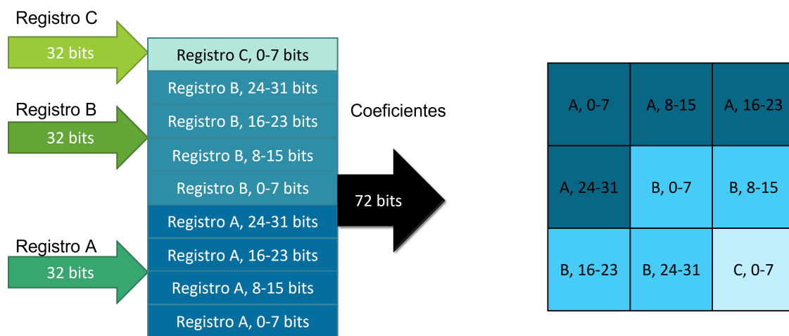
Figura 3-7.: Representaciones del kernel 3x3 a nivel de registros (izquierda) y a nivel de matriz (derecha).
