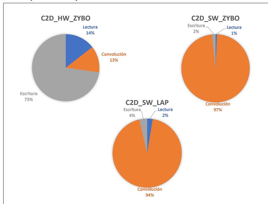
Figura 4-11.: Tiempos acumulados de los métodos para realizar la convolución 2D.
