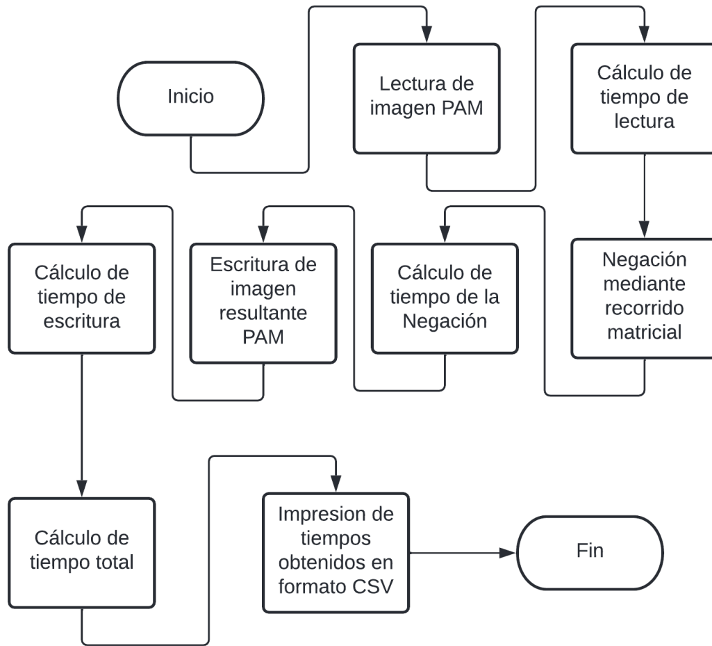
Figura 3-18.: Diagrama de flujo del software de la negación solo por software.
