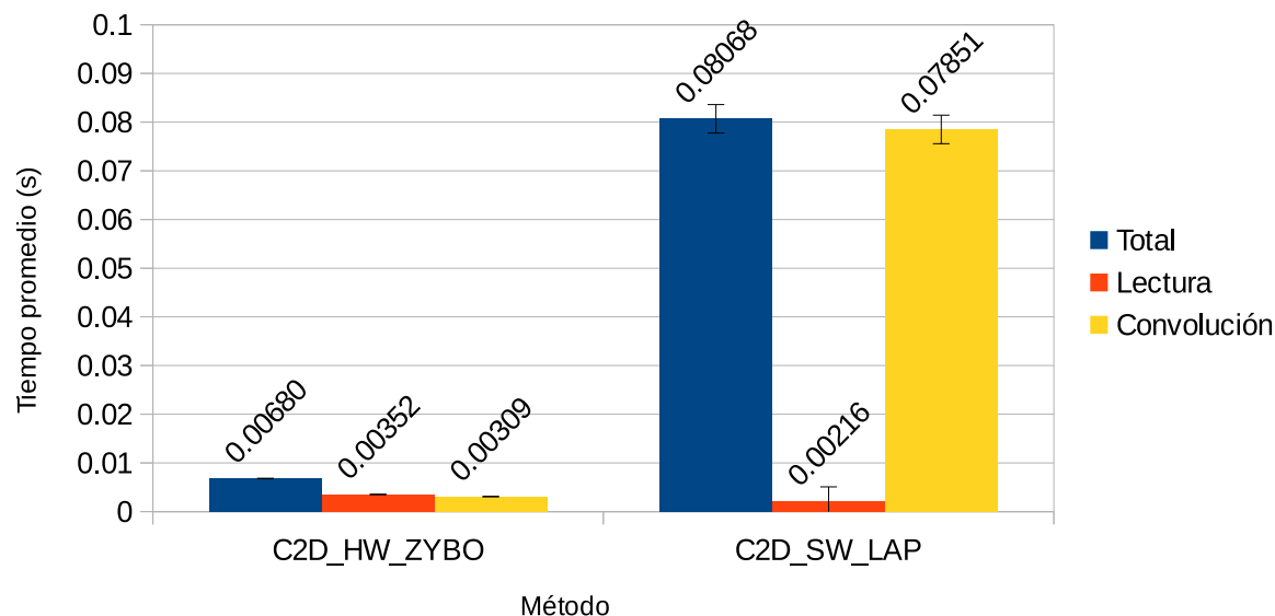
Figura 4-9.: Tiempos promedios para la convolución 2D en dos métodos sin la escritura.
