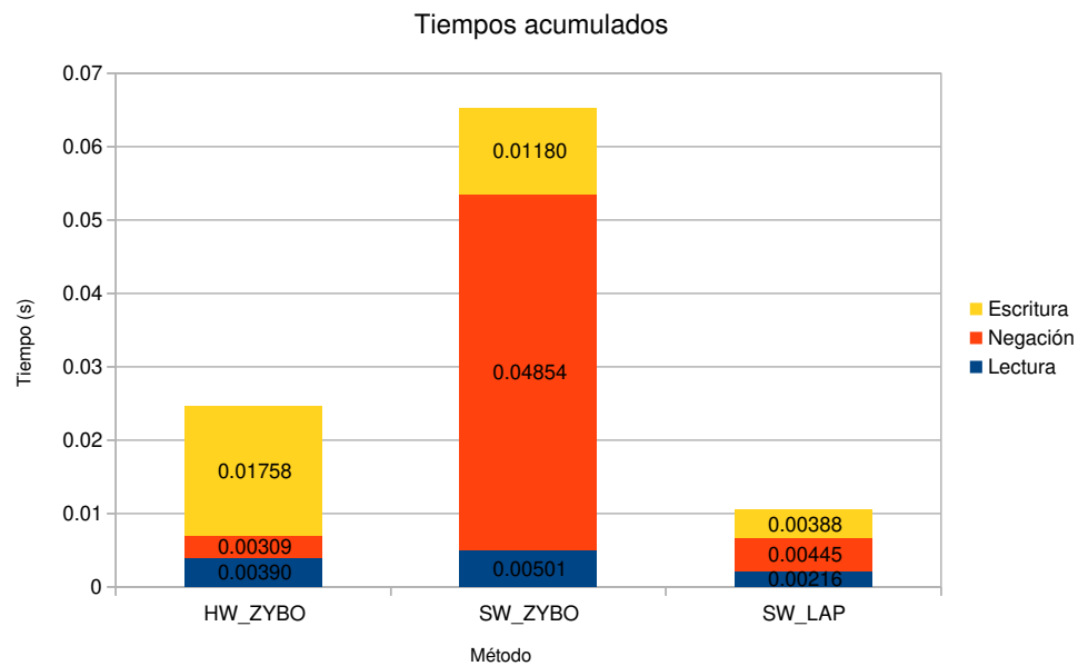
Figura 4-3.: Tiempos acumulados de la negación.
