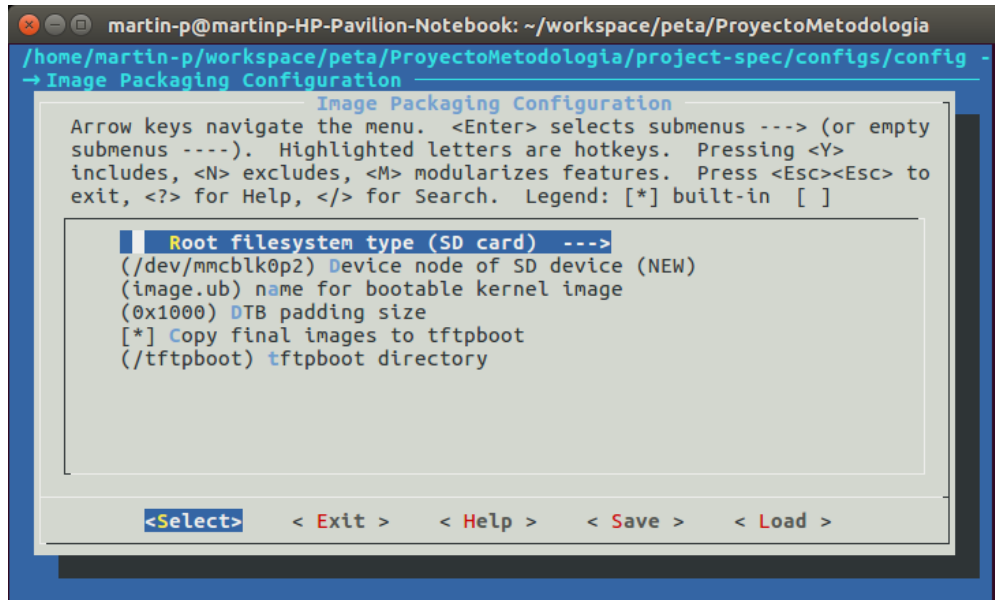
Figura A-3.: Selección del sistema de archivos sobre la microSD.
