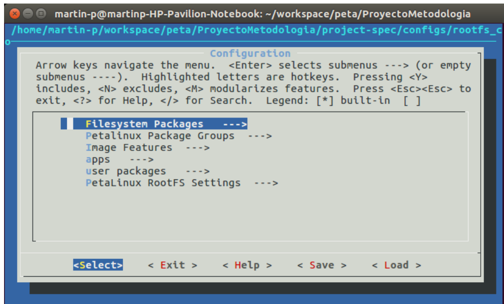
Figura A-4.: Configuración del sistema de archivos.
