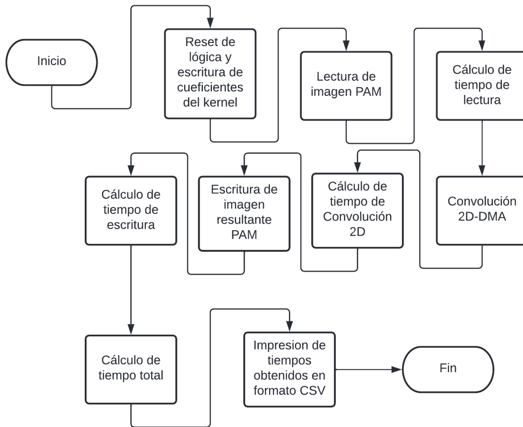
Figura 3-17.: Diagrama de flujo del software de interfaz de la convolución 2D por hardware.
