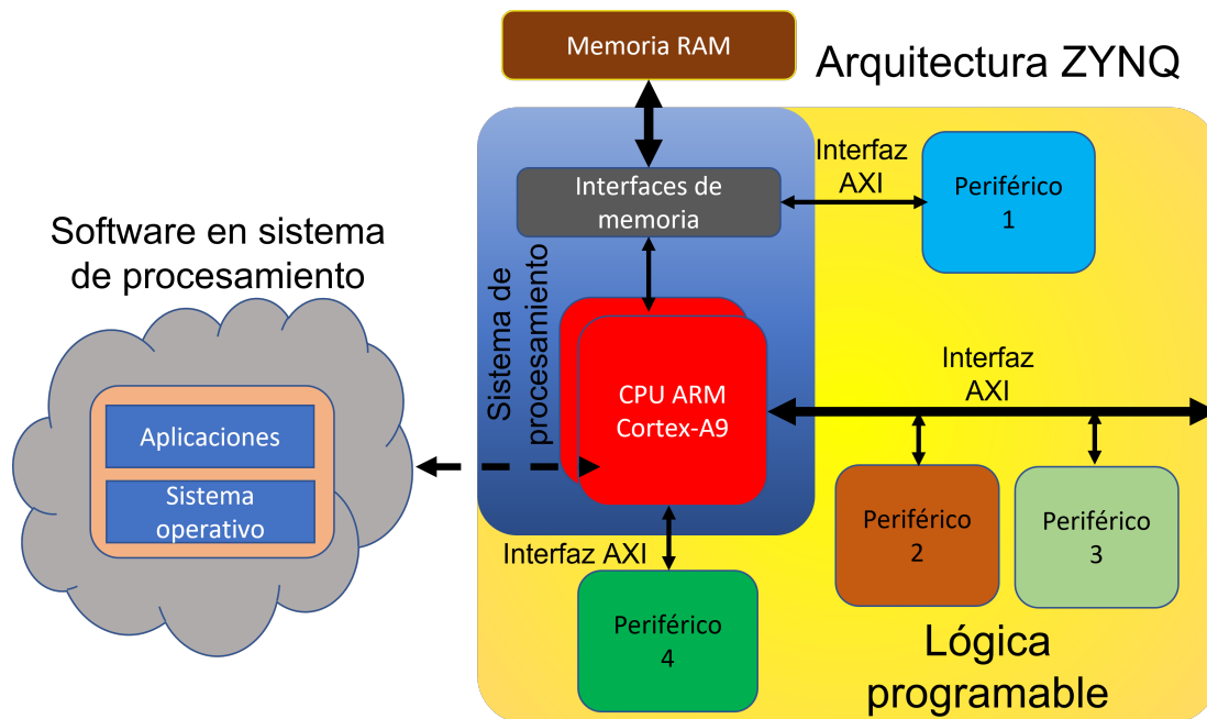
Figura 2-3.: Diagrama simplificado de la arquitectura ZYNQ [7]
