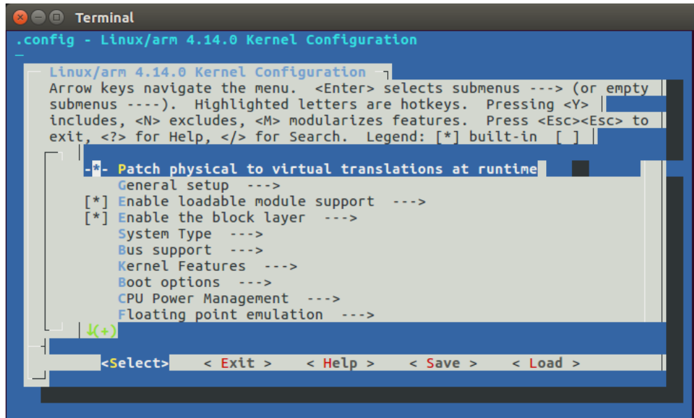
Figura A-6.: Ventana de configuración del kernel.
