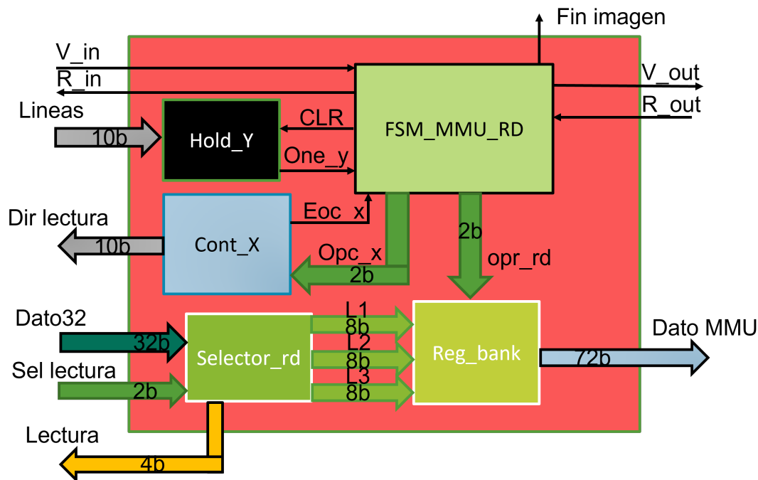
Figura 3-13.: Bloque MMU RD.
