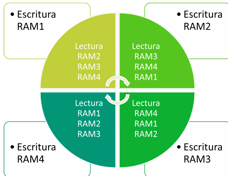
Figura 3-12.: Orden de selección de registros por parte del Selector_w.
