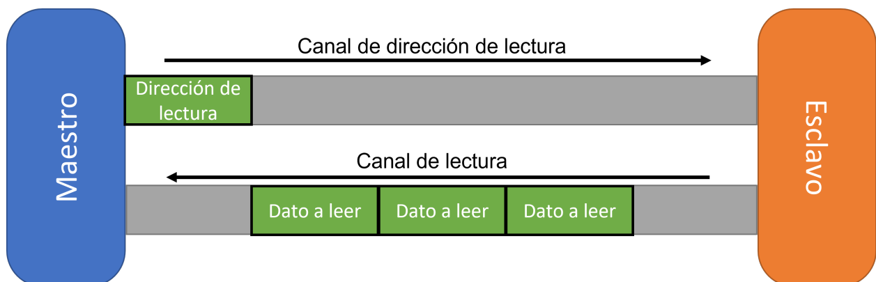
Figura 2-5.: Arquitectura AXI para lectura [7]
