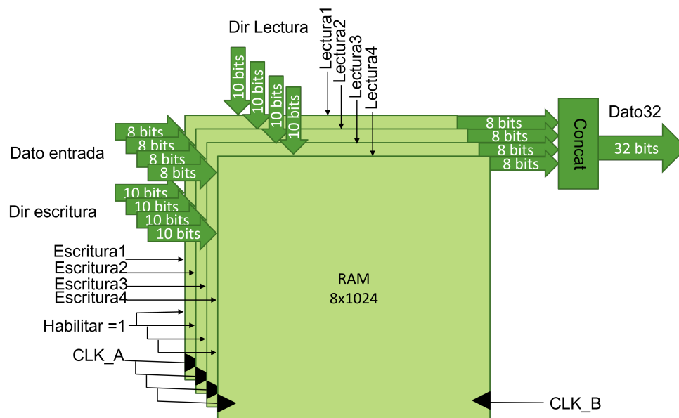
Figura 3-10.: Bloque compuesto por 4 BRAMS.
