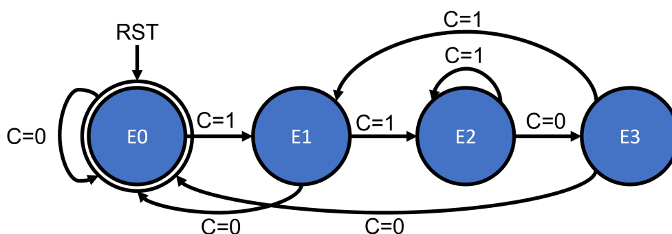
Figura 2-8.: Ejemplo de un diagrama de una máquina de estados finitos.
