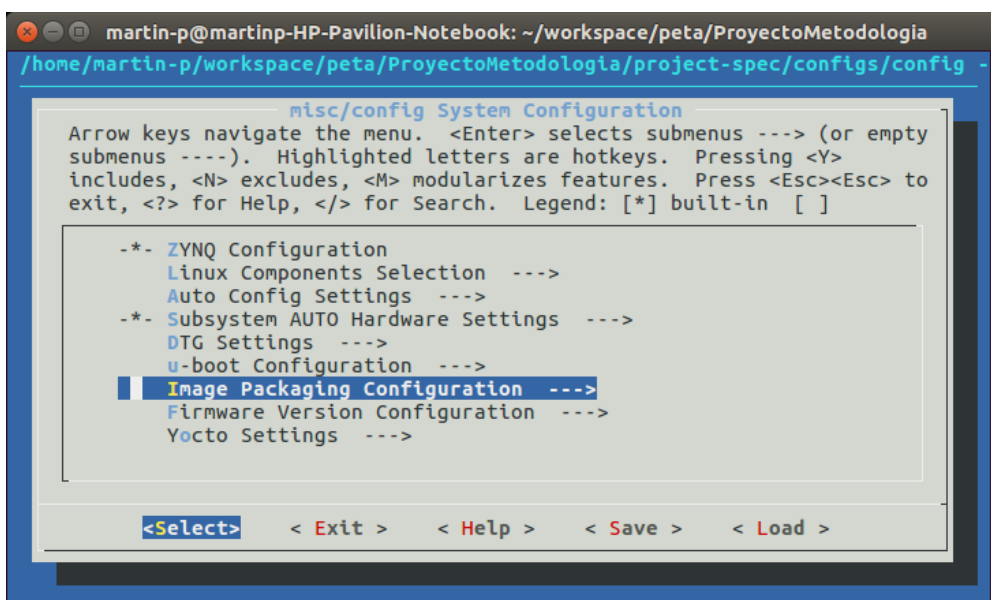
Figura A-2.: Ventana de selección de opciones de empaquetado.
