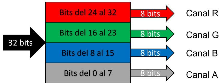
Figura 3-5.: Diagrama del separador de canales.
