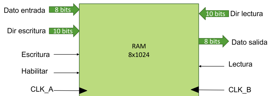
Figura 3-9.: Dual Port RAM.
