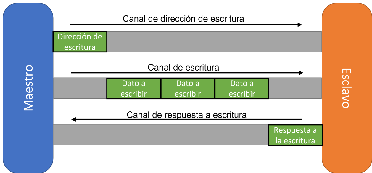
Figura 2-4.: Arquitectura AXI para escritura [7]
