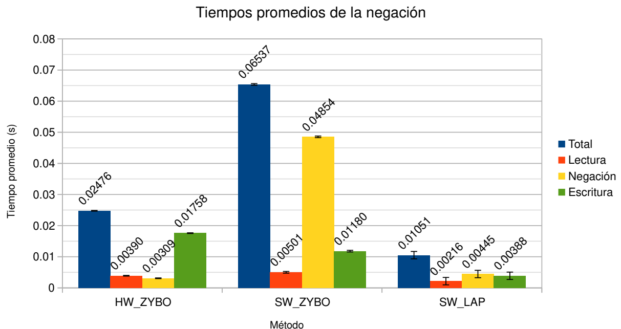
Figura 4-1.: Tiempos promedios al implementar los tres métodos para realizar la negación.
