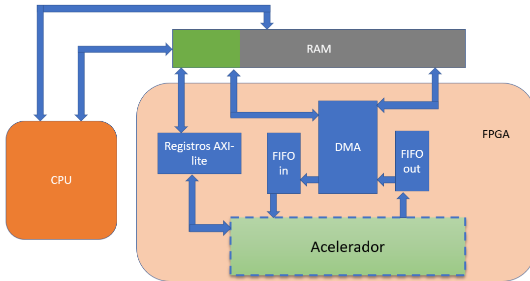
Figura 3-2.: Hardware base de esta investigación.
