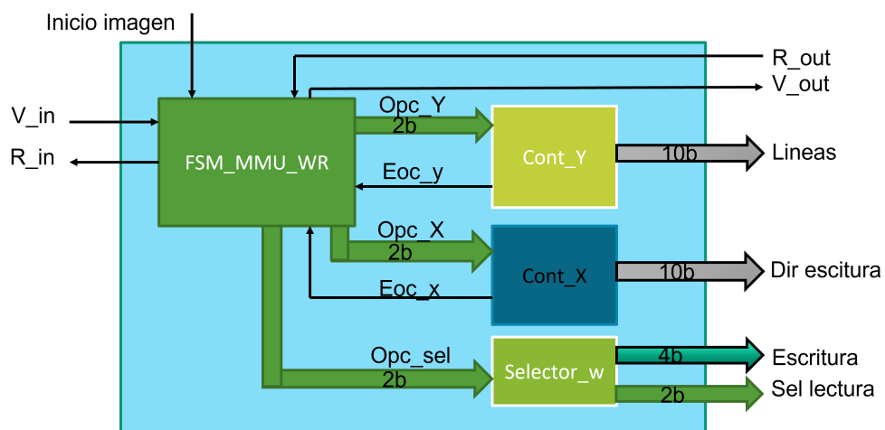
Figura 3-11.: Bloque MMU WR.
