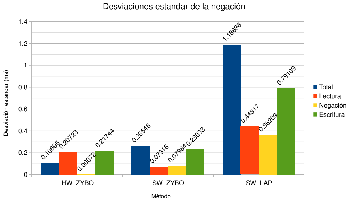
Figura 4-2.: Desviación estándar del tiempo necesario para calcular la negación.
