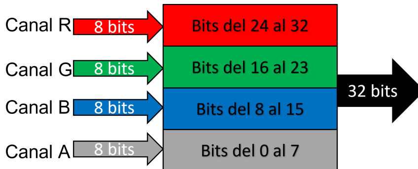
Figura 3-6.: Diagrama del concatenador de canales.
