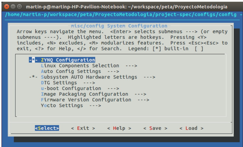
Figura A-1.: Ventana inicial de configuración de Petalinux.
