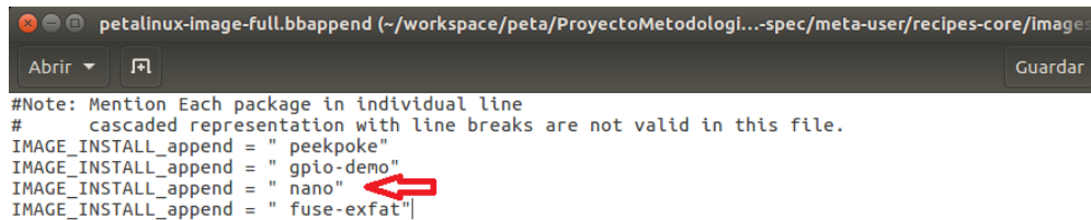
Figura A-5.: Modificación de archivo de configuración para incluir “nano”.
