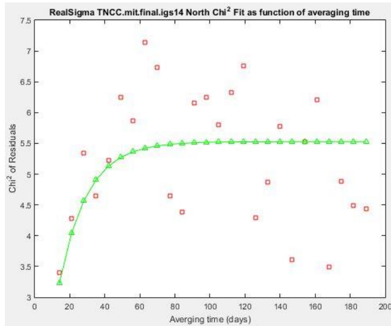
Figura 65. Ajuste exponencial de los valores de \chi^2/\text{gl} de los residuos en el promedio temporal de estación TNCC de la componente norte.
