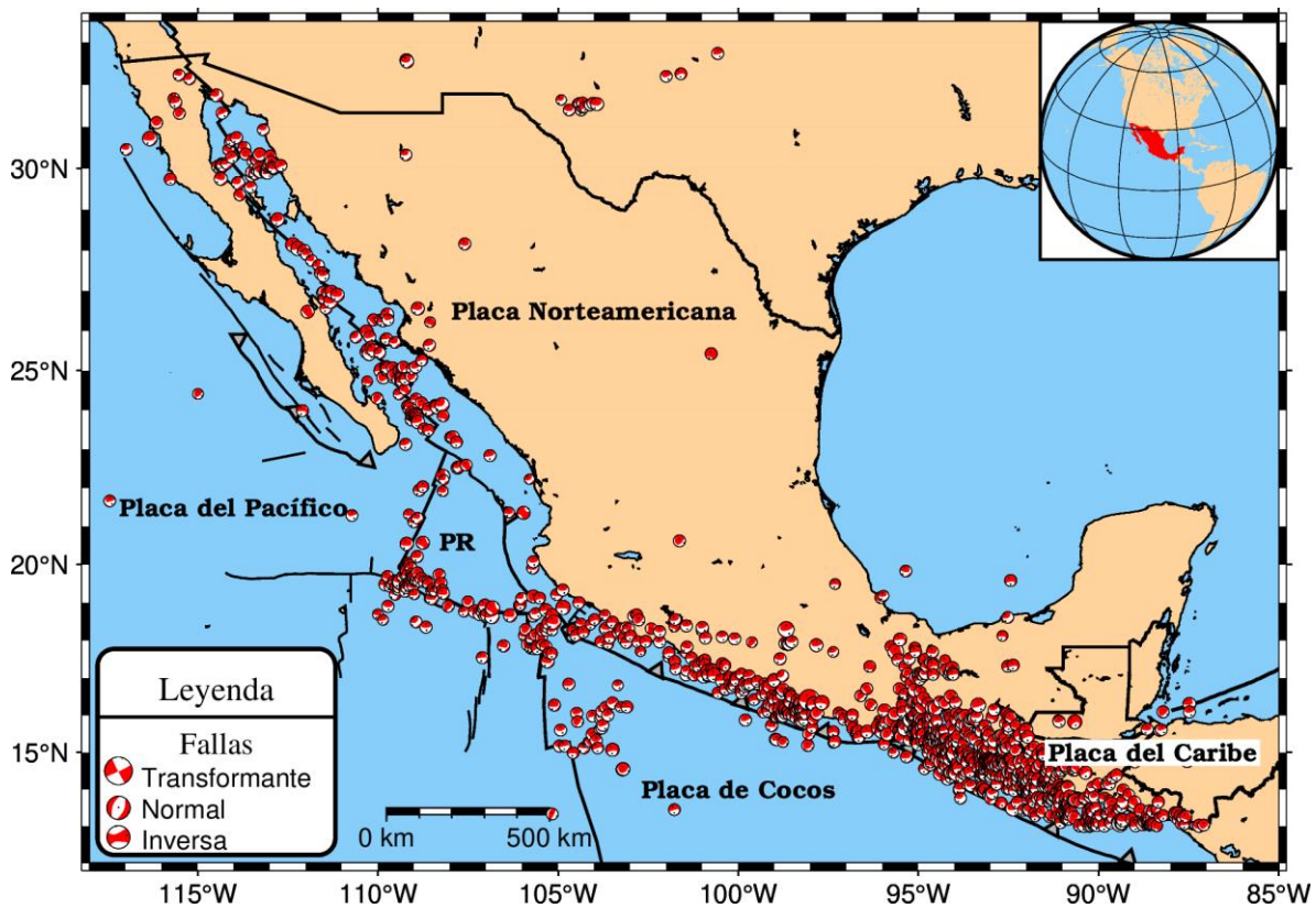
Figura 2. Mecanismos focales del occidente y sur de México. Datos proporcionados por el SSN. PR: Placa de Rivera. El mapa se realizó a través del programa GMT (Wessel et al., 2013).
