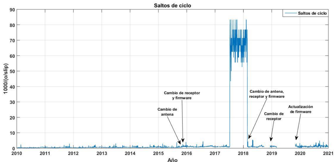
Figura 34. Saltos de ciclo de la estación PENA en el periodo de estudio.
