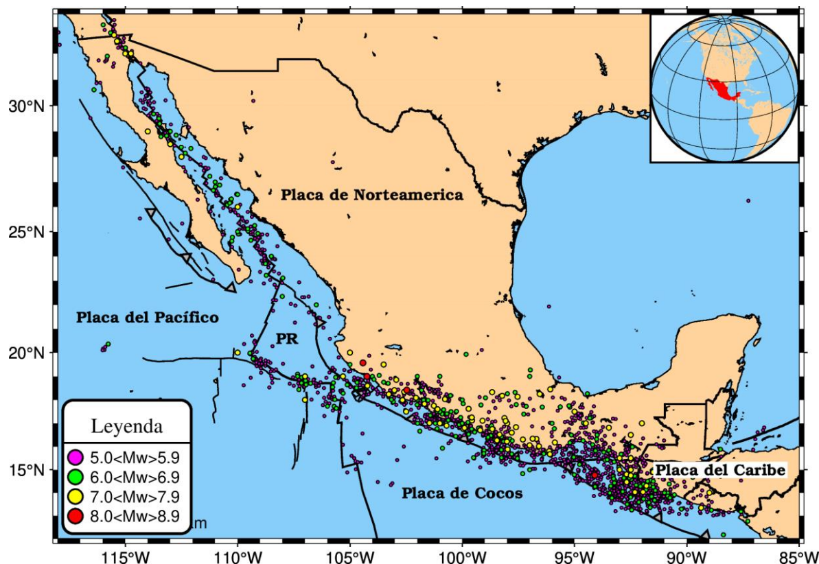
Figura 1. Sismicidad en México. Creado a partir de datos del Servicio Sismológico Nacional (SSN, 2023) con sismos M_w \geq 5 desde 1900 hasta abril del 2021. PR: Placa de Rivera. El mapa se realizó a través del programa GMT (Wessel et al., 2013).
