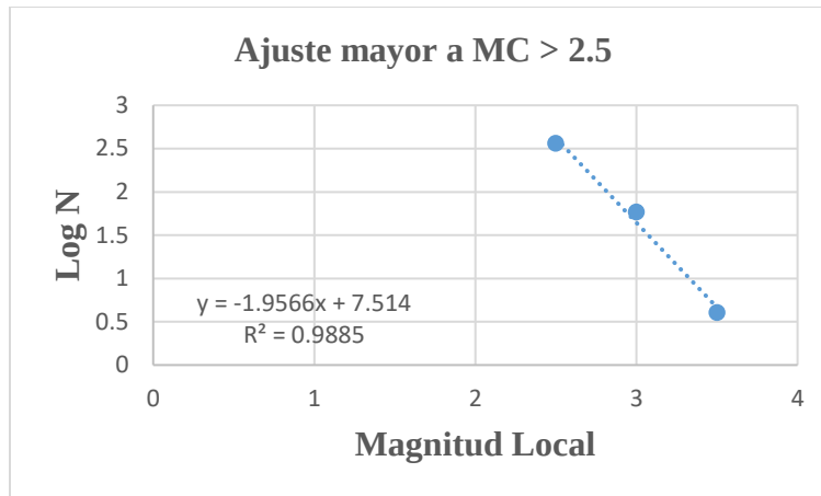
Figura 95. Estimación en Excel del valor de b.
