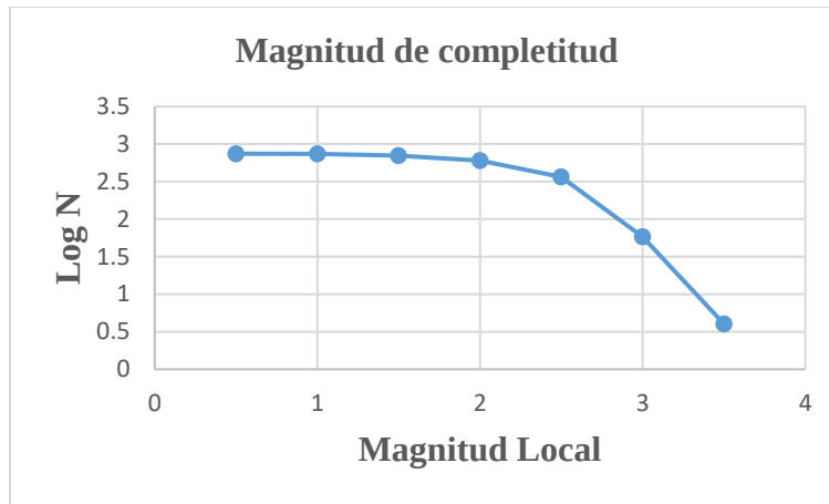
Figura 93. Estimación manual de la magnitud de completitud.
