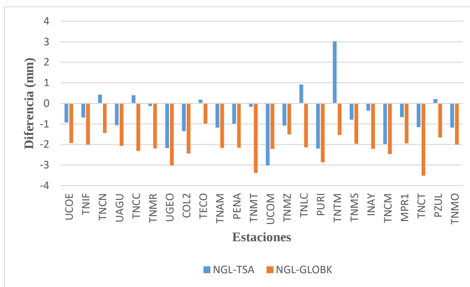
Figura 69. Residuales de velocidad entre NGL-tsviiew y NGL-GLOBK de la componente este.
