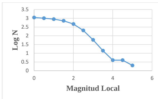
Figura 75. Estimación manual de la magnitud de completitud.
