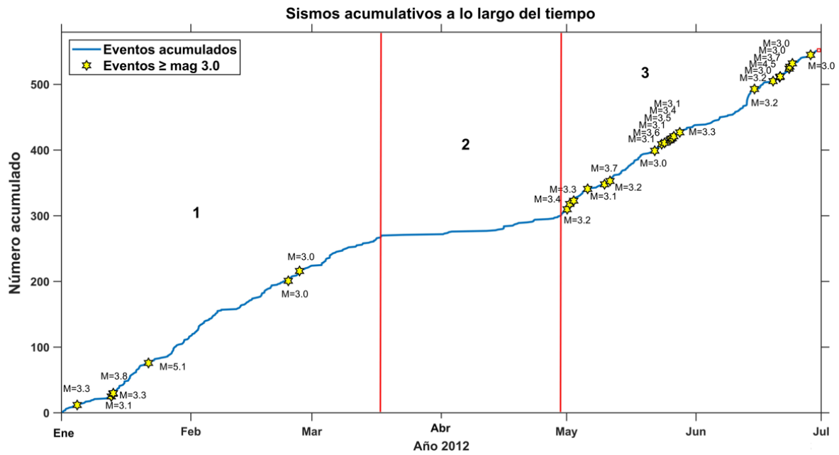
Figura 77. Número acumulativo de sismos.
