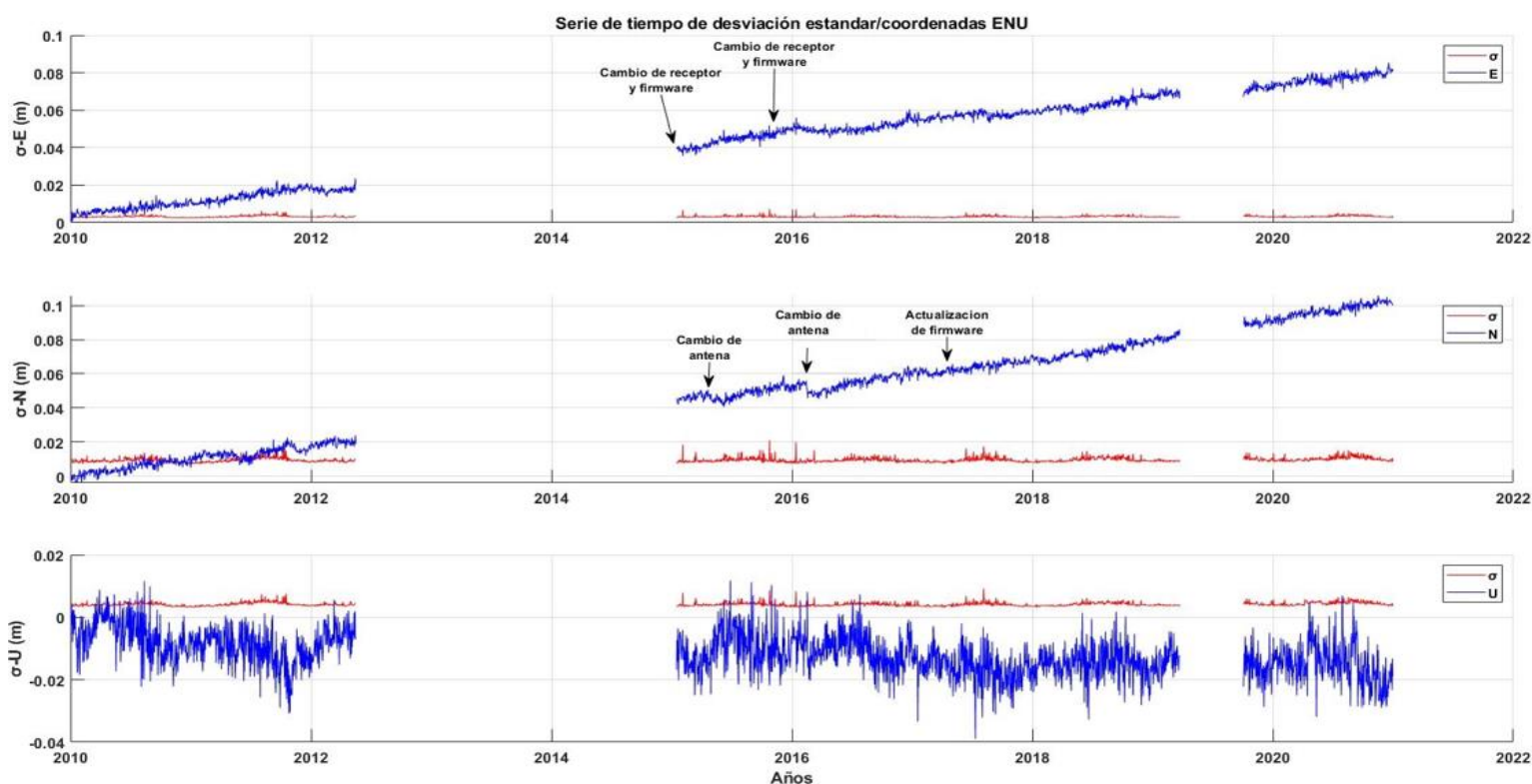
Figura 46. Serie de tiempo de coordenadas ENU y desviación estándar de estación TECO
