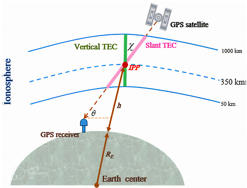
Figura 2.2: La figura muestra la geometría entre un satélite GPS y un receptor en la Tierra para medir el TEC. El STEC es el TEC medido en la trayectoria oblicua del satélite al receptor, mientras que el VTEC es el TEC proyectado verticalmente. El ángulo de elevación ( \theta ) y el Punto de Penetración Ionosférica (IPP) permiten corregir el STEC para calcular el VTEC, proporcionando una medición vertical precisa del TEC en la ionosfera. Fuente: Thai GNSS and Space Weather Information Data Center (2023).
