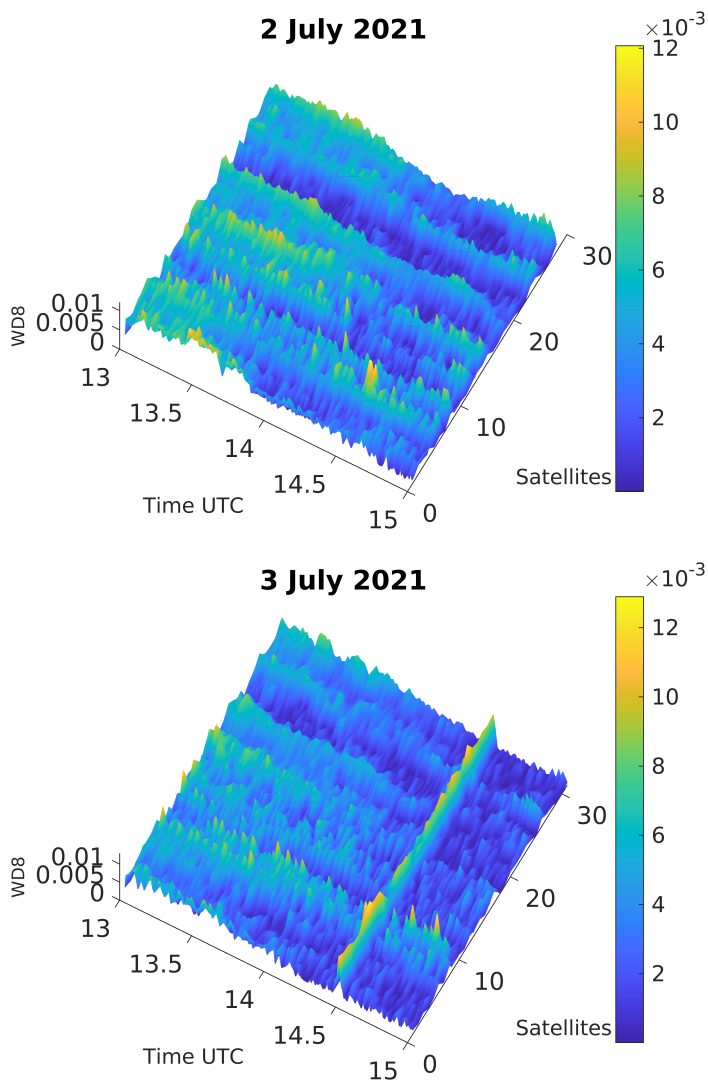
Figura 4.2: Comparación entre un día calmado (2 de julio de 2021, imagen superior) y el evento del 3 de julio de 2021 (imagen inferior). Se observan fluctuaciones más intensas en el evento del 3 de julio, destacadas por mayores valores en la escala de colores, lo que indica un aumento significativo en la actividad. Los gráficos muestran el comportamiento de la relación VTEC con el número de satélites, donde los picos más pronunciados el día del evento reflejan posibles perturbaciones ionosféricas relacionadas con la actividad observada.
