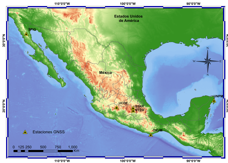
Figura 3.1: Mapa de distribución de las estaciones GNSS de la Red de la UNAM, utilizadas en el cálculo del TEC para el análisis de la ionosfera. Estas estaciones están ubicadas de manera que permiten una cobertura adecuada de la región, proporcionando datos clave para monitorear variaciones ionosféricas y su relación con los eventos.
