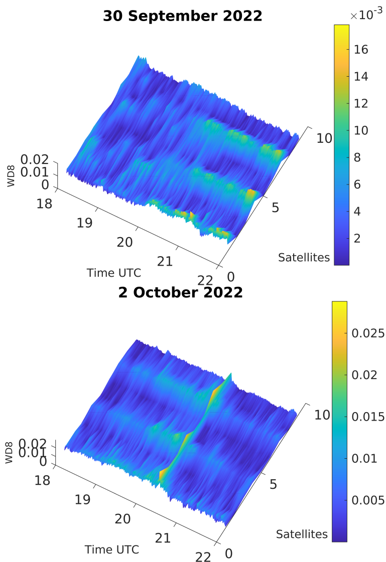
Figura 4.31: Comparación entre el día calmado (30 de septiembre de 2022, imagen superior) y el evento del 2 de octubre de 2022 (imagen inferior). El evento del 2 de octubre muestra fluctuaciones marcadas, con picos elevados en la escala de colores, lo que indica una perturbación ionosférica frente al comportamiento estable del día anterior. Las variaciones del VTEC en función del número de satélites destacan el impacto del evento.
