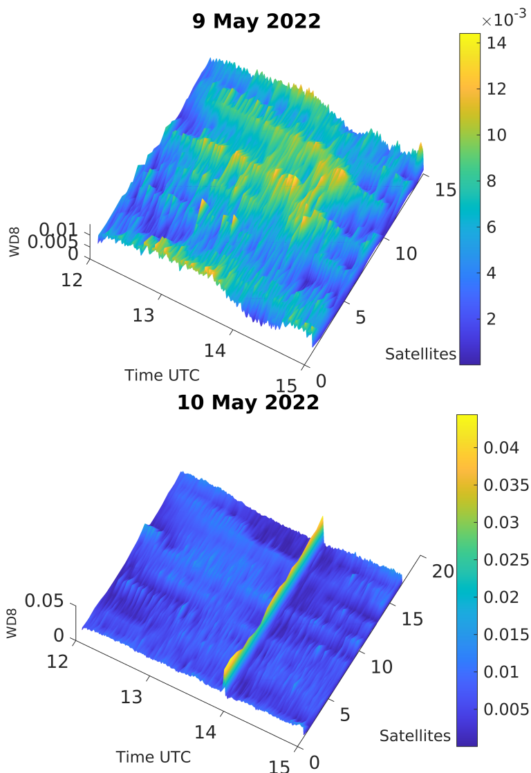
Figura 4.25: Comparación entre un día tranquilo (9 de mayo de 2022, imagen superior) y el evento del 10 de mayo de 2022 (imagen inferior). El evento del 10 de mayo muestra fluctuaciones más pronunciadas, con picos elevados en la escala de colores, indicando una perturbación ionosférica en comparación con el día previo. Se destacan las variaciones del VTEC en función del número de satélites, reflejando el impacto del evento.
