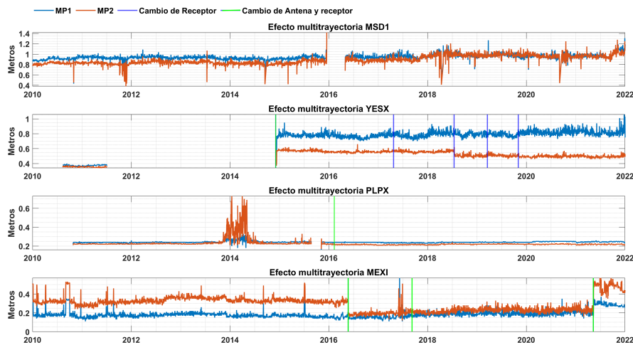
FIGURA 4.3: Series temporales de multitrayectoria y actualizaciones de antena y receptor en las estaciones MSD1, YESX, PLPX y MEXI.
