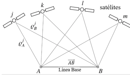
FIGURA 2.2: Concepto de posicionamiento relativo. Fuente: (Hofmann-Wellenhof, B., Lichtenegger, H., y Wasle, 2008).
