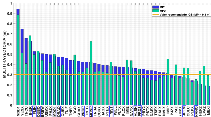
FIGURA 4.2: Promedio global de efecto multitrayectoria por estación: MP1 y MP2. La línea amarilla muestra el valor máximo recomendable por el IGS para la cantidad de efecto multitrayectoria. Las estaciones dentro del recuadro azul pertenecen al marco de referencia.
