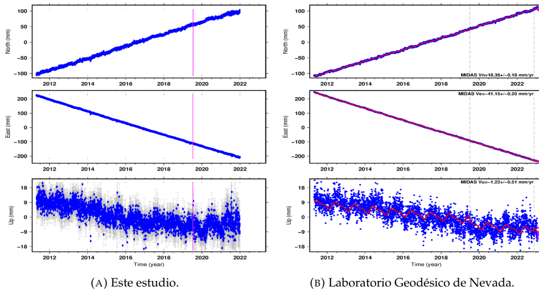
FIGURA 4.11: Comparativa de series temporales de la estación PTEX relativas al marco ITRF14.
