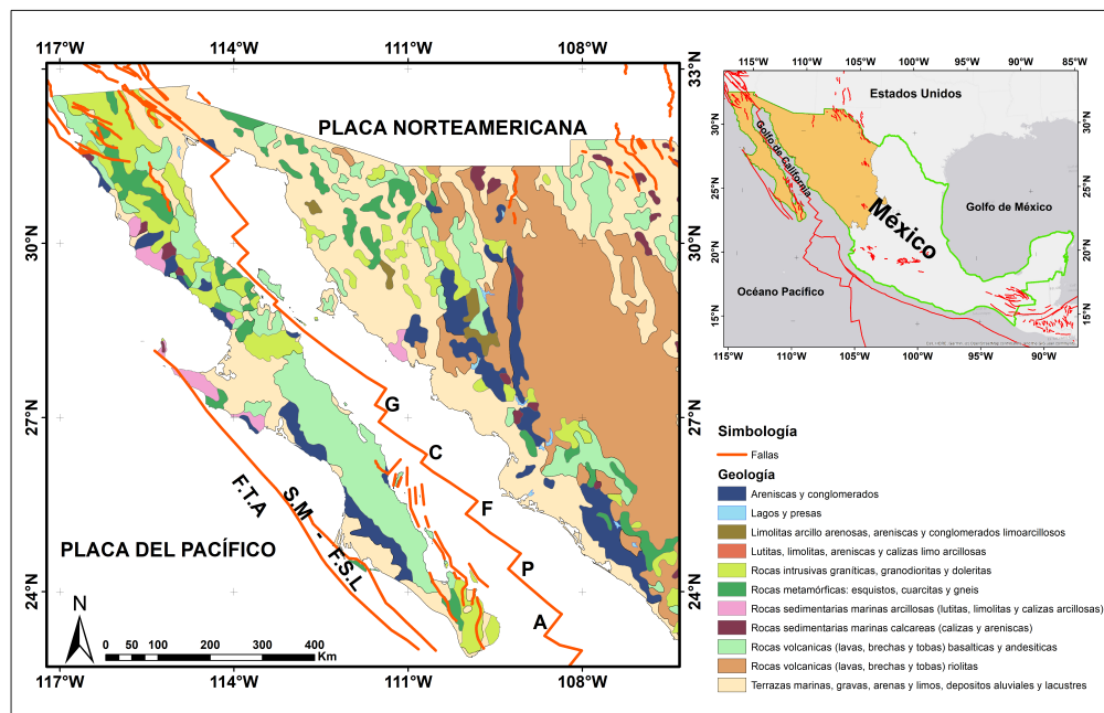
FIGURA 1.1: Mapa Geológico del Noroeste de México, datos geológicos de INEGI (2021). Centros de Dispersión (Ferrari y col., 2013): G-Guaymas, C-Carmen F-Fallarón P-Pescadero A-Alarcón. F.T.A-Falla Tosco Abreojos, S.M-F.S.L - Fallas Santa Margarita-Falla San Lorenzo.
