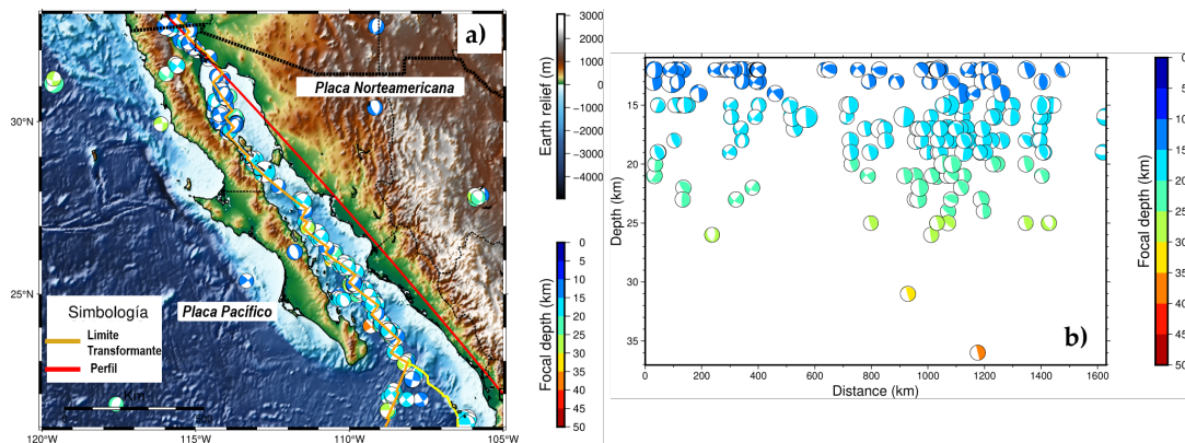
FIGURA 1.3: a) Mecanismos focales de la actividad sísmica en el Golfo de California, México en el periodo 2010-2022. b) Profundidad de los hipocentros del perfil indicado en la Figura a.
