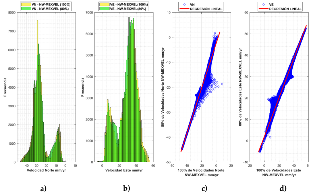
FIGURA 4.31: Validación directa punto a punto del modelo generado con el 80 % de las velocidades conocidas respecto al modelo generado con el 100 % de velocidades conocidas. a) Histograma de velocidad en la componente Norte. b) Histograma de velocidad en la componente Este. c) Correlación entre las componentes Este-Este. d) Correlación entre las componentes Norte-Norte.
