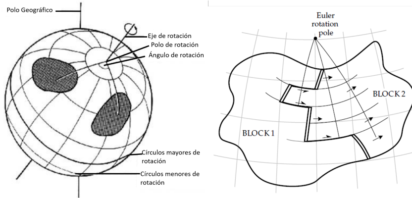
FIGURA 2.3: Diagrama de Rotación del polo de Euler.
