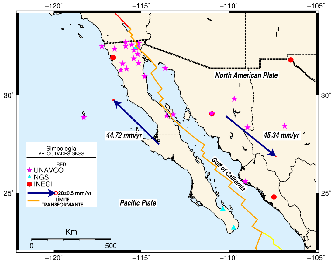
FIGURA 4.19: Velocidades horizontales promedio para la Placa Norteamericana (relativa a la Placa Pacífico) y la Placa del Pacífico (relativa a la Placa Norteamericana).
