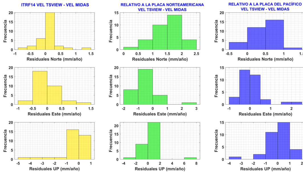
FIGURA 4.16: Velocidades residuales entre la estimación con TSVIEW y MIDAS de las 33 estaciones GPS relativas al marco de referencia ITRF14, Placa Norteamericana y relativa a la Placa del Pacífico.
