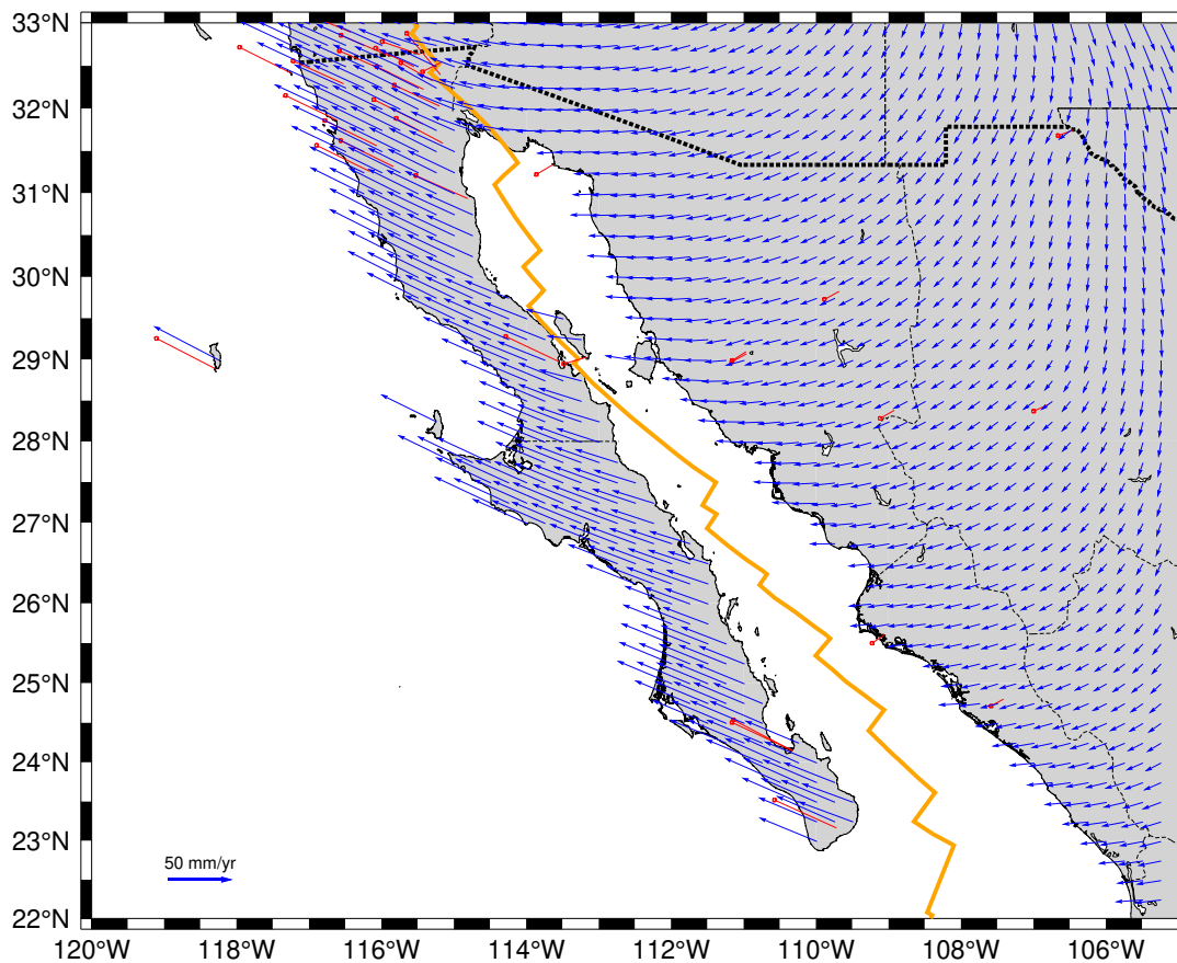
FIGURA 4.22: Modelo NW-MEXVEL de Velocidades horizontales interpoladas mediante funciones de Green con un coeficiente de Poisson de 0.5 considerando acoplamiento elástico. Vectores rojos: velocidades obtenidas del procesamiento en GAMIT/GLOBK. Vectores azules: Velocidades interpoladas en un grid de 15' X 15' de arco.
