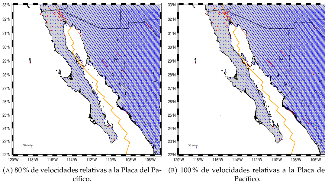
FIGURA 4.26: Modelo de Velocidades horizontales respecto a la Placa del Pacífico, interpoladas mediante funciones de Green con un coeficiente de Poisson de 0.5 considerando acoplamiento elástico. Vectores rojos: velocidades obtenidas del procesamiento en GAMIT/GLOBK. Vectores azules: Velocidades interpoladas en un grid de 15' x 15' de arco.
