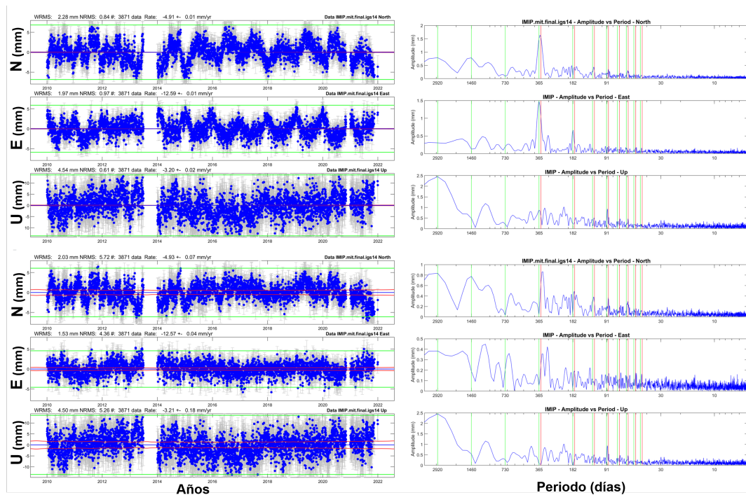
FIGURA 4.14: Series temporales de la estación IMIP, con (inferior) y sin (superior) considerar efecto anual y semianual. A la derecha el espectro de frecuencia correspondiente.
