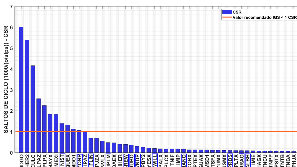
FIGURA 4.5: Promedio global de los saltos de ciclo por cada mil observaciones por estación. Las estaciones dentro del recuadro azul pertenecen al marco de referencia.
