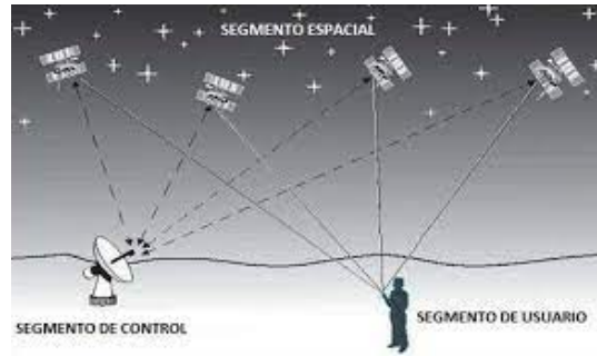
FIGURA 2.1: Segmento espacial, control y usuario en los GNSS.
