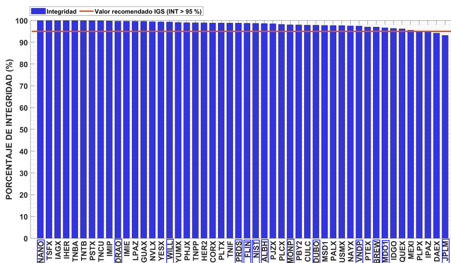
FIGURA 4.6: Promedio global de integridad por estación. Las estaciones dentro del recuadro azul pertenecen al marco de referencia.
