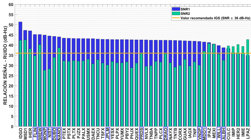
FIGURA 4.4: Promedio global de la relación señal-ruido por estación: SNR1 y SNR2. Las estaciones dentro del recuadro azul pertenecen al marco de referencia.
