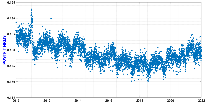
FIGURA 4.8: Valores del nrms del postfit de las soluciones diarias obtenidas en GAMIT para los 12 años.
