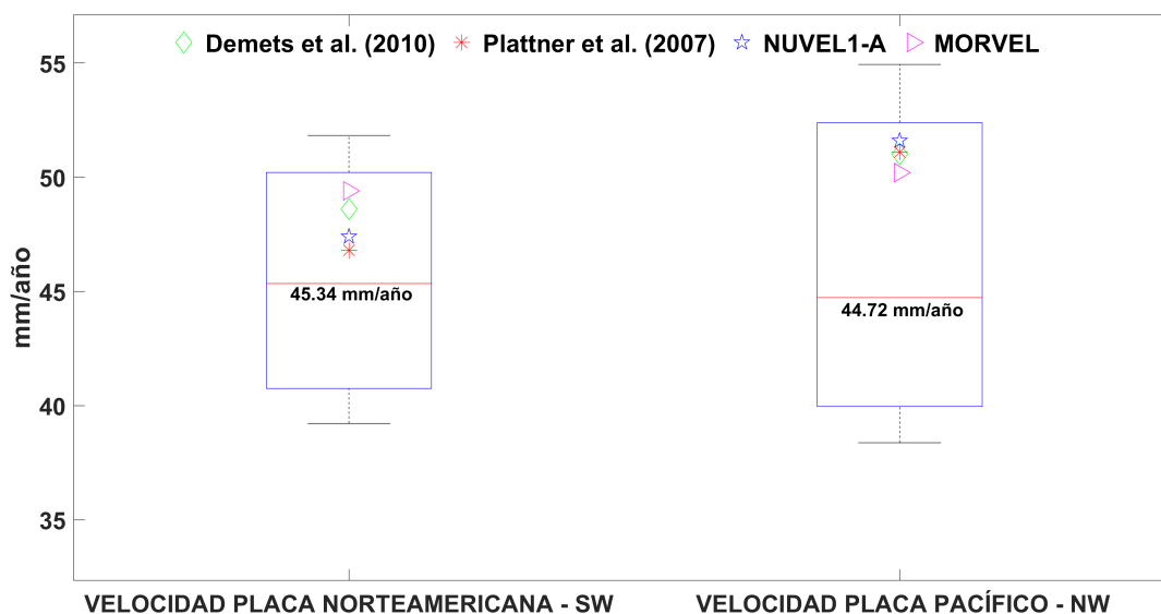
FIGURA 4.20: Velocidades horizontales para cada placa tectónica reportadas en el estado del arte. El diagrama de caja y bigote muestra el resultado de este estudio.
