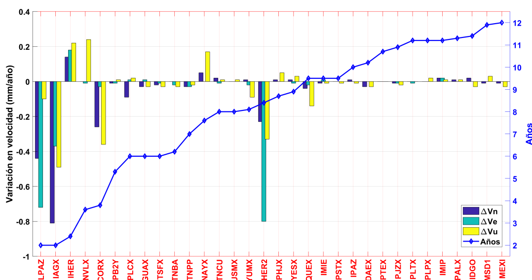
FIGURA 4.15: Diferencias entre las componentes de velocidad con y sin señales estacionales y su relación con el tiempo de operación continua.
