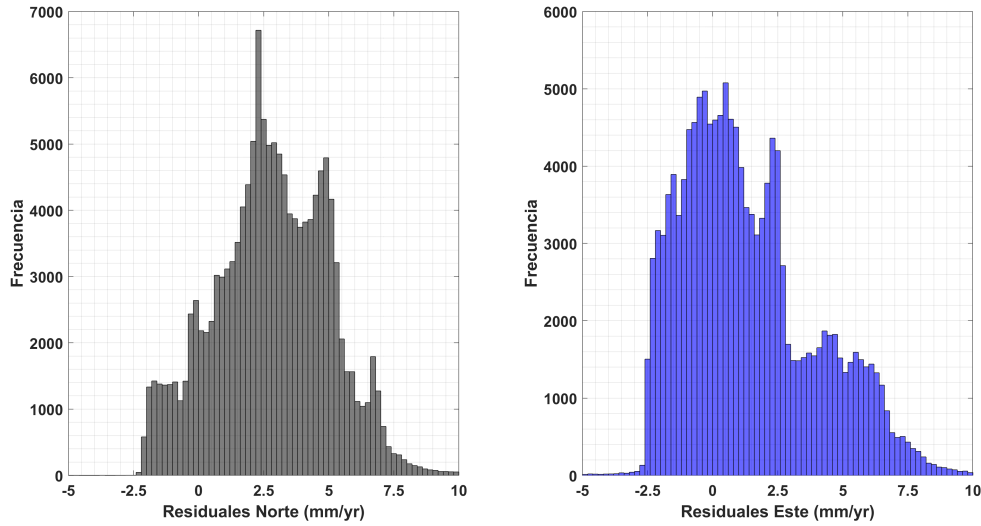
FIGURA 4.24: Residuales horizontales del modelo NW-MEXVEL (este estudio) tomando como referencia las velocidades interpoladas por el modelo GEODVEL 2010.
