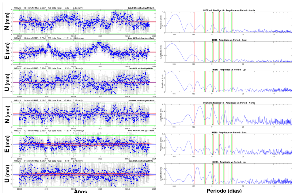
FIGURA 4.12: Series temporales de la estación IHER, con (inferior) y sin (superior) considerar efecto anual y semianual. A la derecha el espectro de frecuencia correspondiente.
