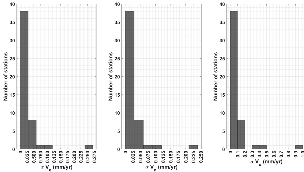
FIGURA 4.10: Desviaciones Estándar de las velocidades calculadas en GLOBK.
