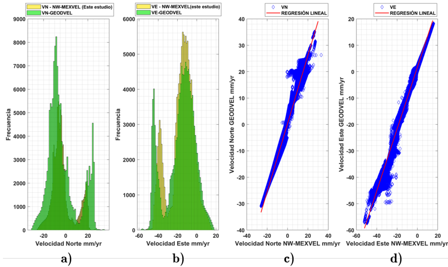
FIGURA 4.25: Validación directa del modelo NW-MEXVEL tomando como referencia el modelo GEODVEL 2010. a) Velocidad en la componente Norte. b) Velocidad en la componente Este. c) Correlación en las componentes Este-Este. d) Correlación en las componentes Norte-Norte.
