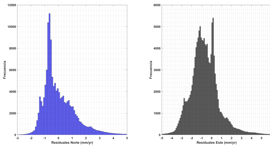
FIGURA 4.30: Residuales horizontales del Modelo NW-MEXVEL relativo a la Placa Norteamericana considerando el modelo generado con el 100 % de las observaciones como modelo de validación.
