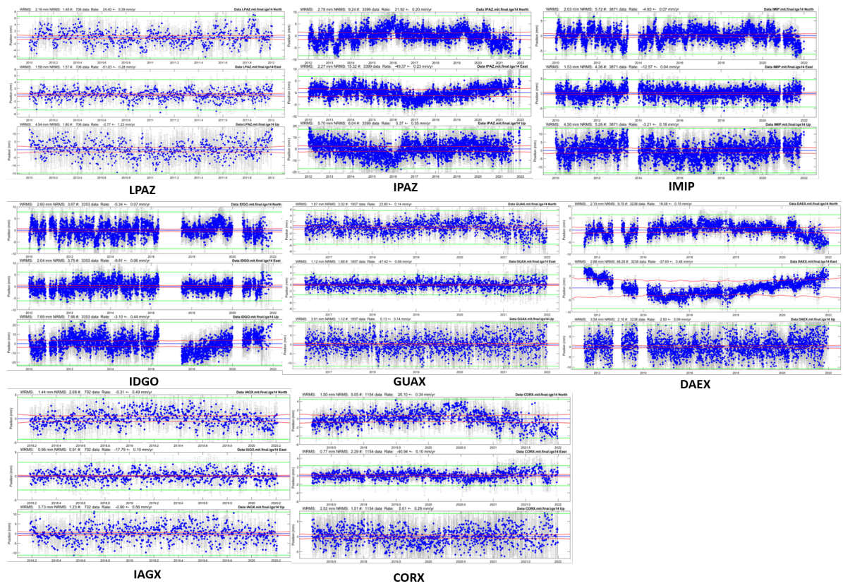
FIGURA A.3: Series temporales analizadas en este estudio con efecto anual y semianual removido ajustadas al marco ITRF14. Estaciones localizadas en el Noroeste de México continuación .
