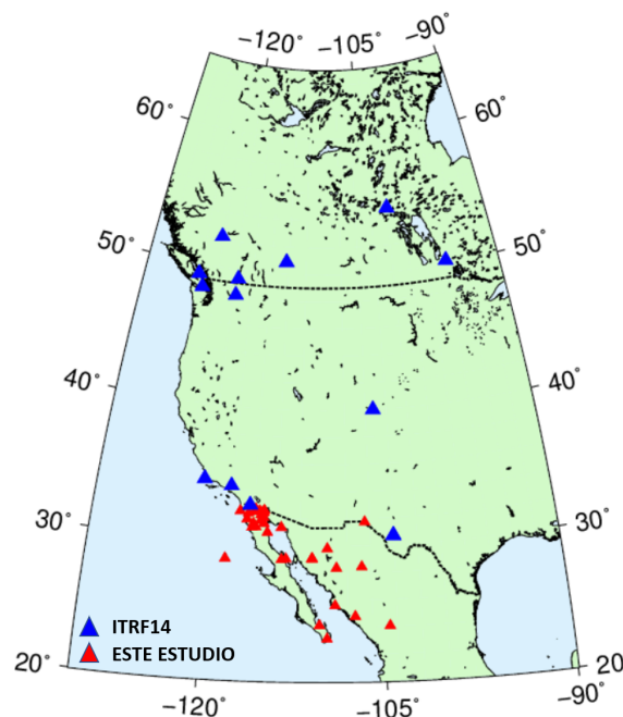
FIGURA 4.7: Localización de estaciones geodésicas para estimación de posicionamiento y velocidades.
