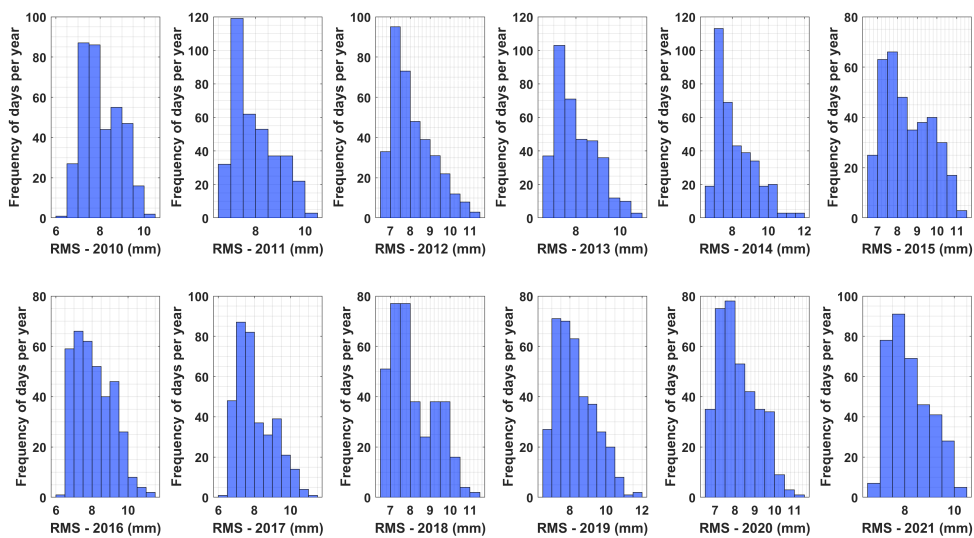
FIGURA 4.9: Raíz cuadrática media ( rms ) de los residuales de fase del procesamiento en GAMIT.
