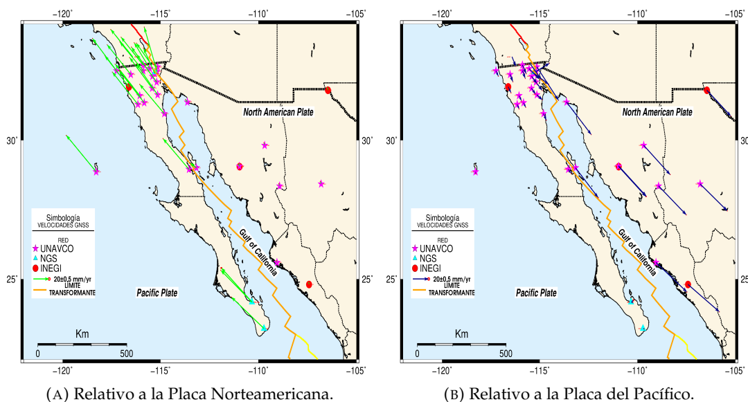
FIGURA 4.18: Velocidades horizontales de estaciones GPS relativas a una placa tectónica.
