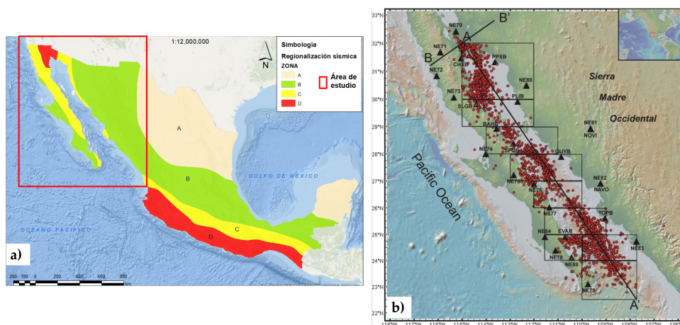
FIGURA 1.2: a) División de Zonas Sísmicas en México (UNAM, 2017). b) Epicentros en el Golfo de California entre 2002 y 2014 (Castro y col., 2017).
