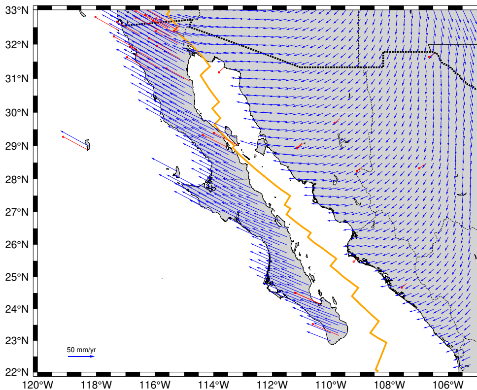
FIGURA 4.23: Modelo de Velocidades horizontales interpoladas mediante funciones de Green con un coeficiente de Poisson de 0.5 considerando acoplamiento elástico. Vectores rojos: Velocidades obtenidas del modelo GEODVEL 2010. Vectores azules: Velocidades interpoladas con funciones de Green (grid 15' X 15' de arco).
