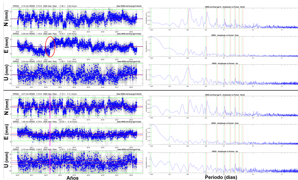
FIGURA 4.13: Series temporales de la estación HER2, con (inferior) y sin (superior) considerar efecto anual y semianual. A la derecha el espectro de frecuencia correspondiente.
