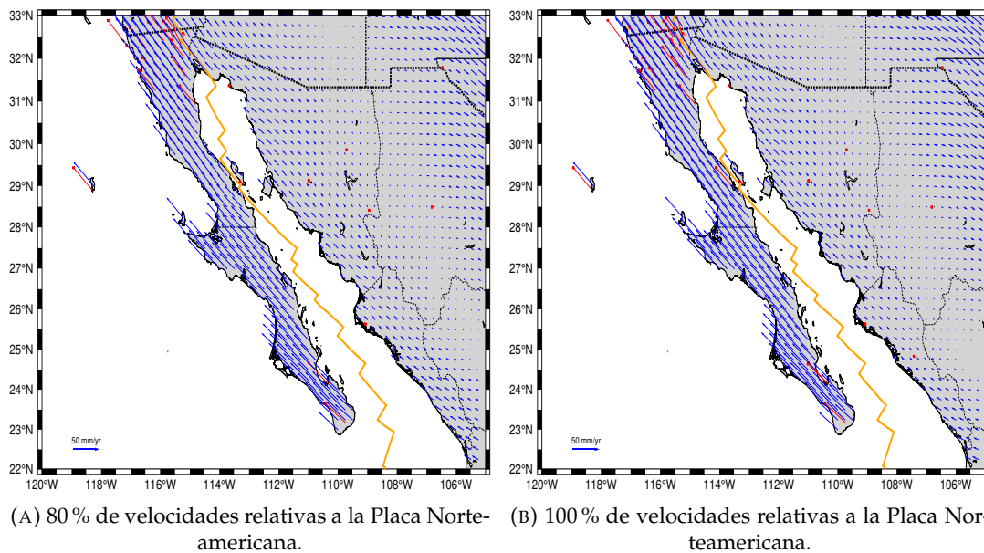
FIGURA 4.29: Modelo de Velocidades horizontales respecto a la Placa Norteamericana, interpoladas mediante funciones de Green con un coeficiente de Poisson de 0.5 considerando acoplamiento elástico. Vectores rojos: velocidades obtenidas del procesamiento en GAMIT/-GLOBK. Vectores azules: Velocidades interpoladas en un grid de 15' \times 15' de arco.
