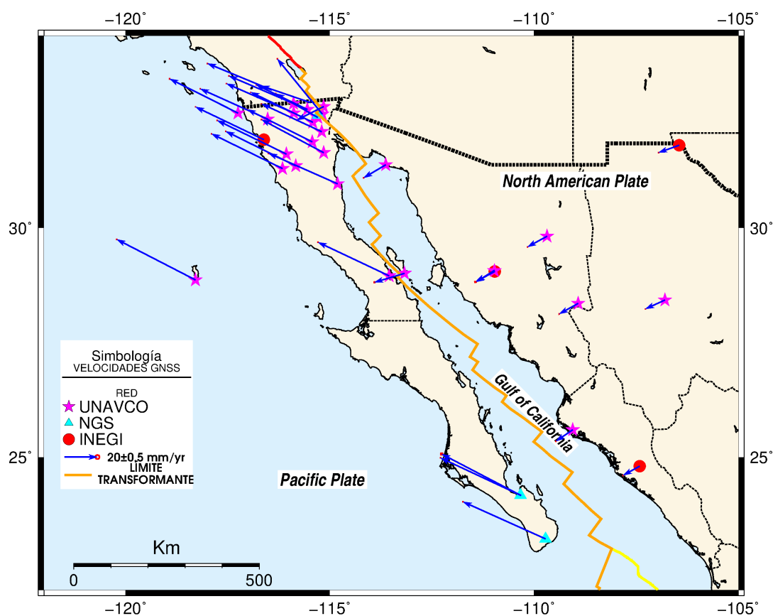
FIGURA 4.17: Velocidades horizontales de estaciones GPS relativas al marco de referencia ITRF14.
