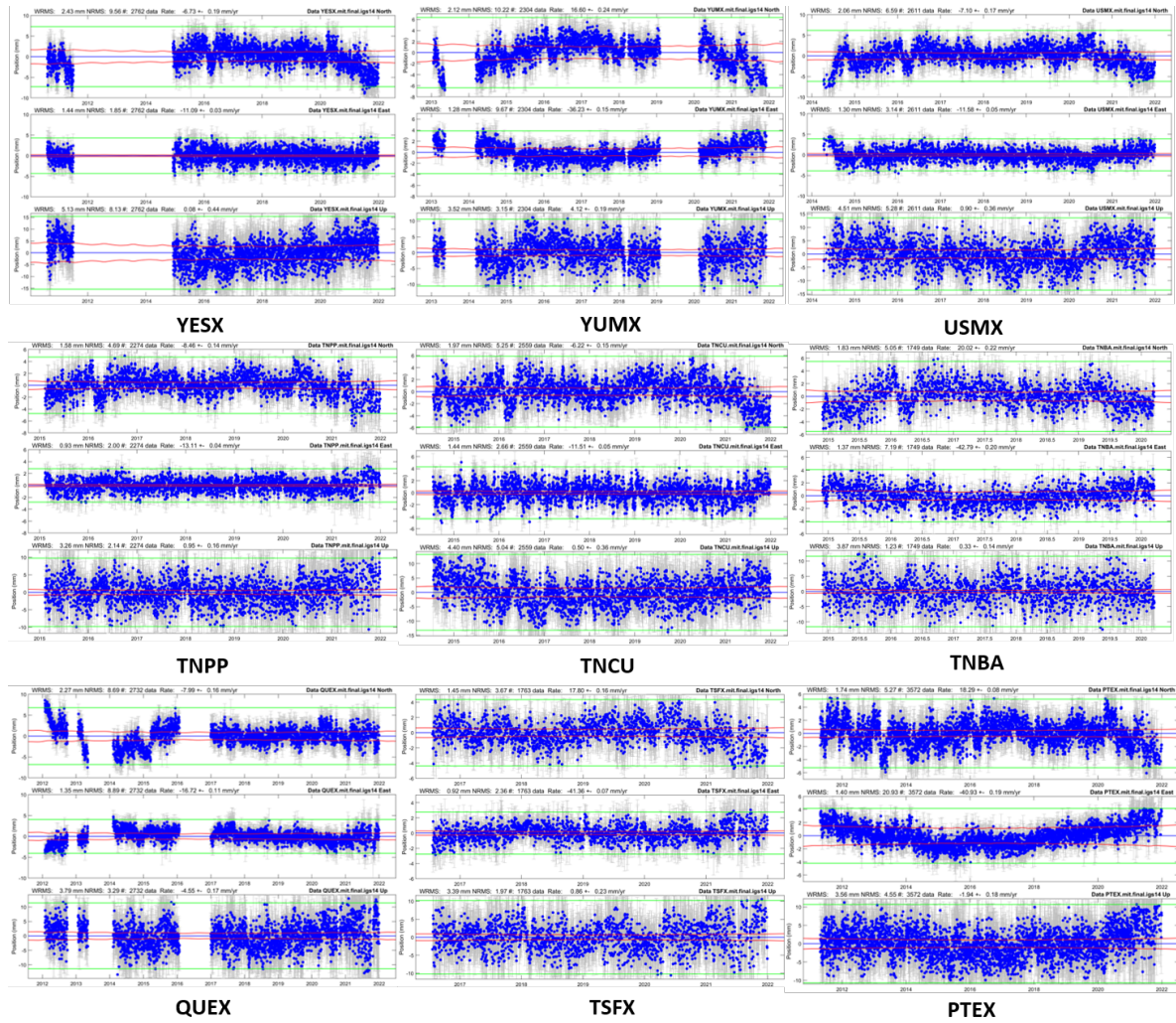
FIGURA A.1: Series temporales analizadas en este estudio con efecto anual y semianual removido ajustadas al marco ITRF14. Estaciones localizadas en el Noroeste de México.
