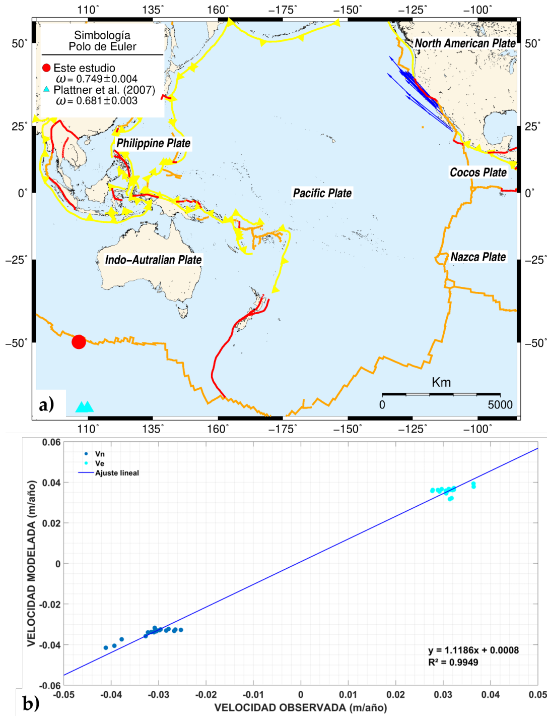
FIGURA 4.21: a) Estimación del polo de Rotación de Euler a través de 18 estaciones en la Península de Baja California. b) Coeficiente de correlación observado vs modelado.
