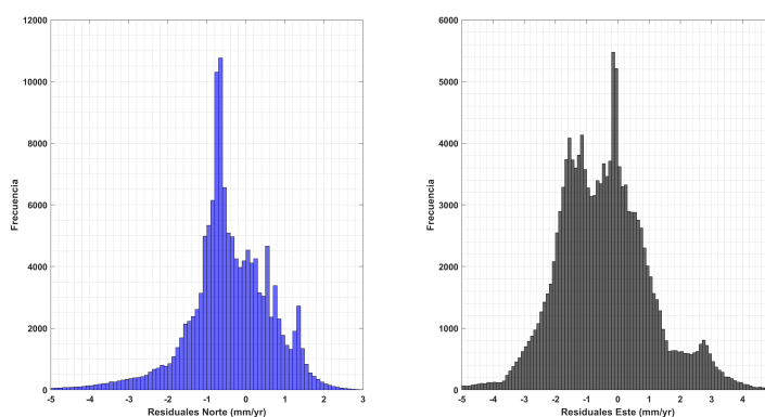
FIGURA 4.27: Residuales horizontales del Modelo NW-MEXVEL relativo a la Placa del Pacífico considerando el modelo generado con el 100 % de las observaciones como modelo de validación respecto al modelo generado con el 80 % de velocidades conocidas.
